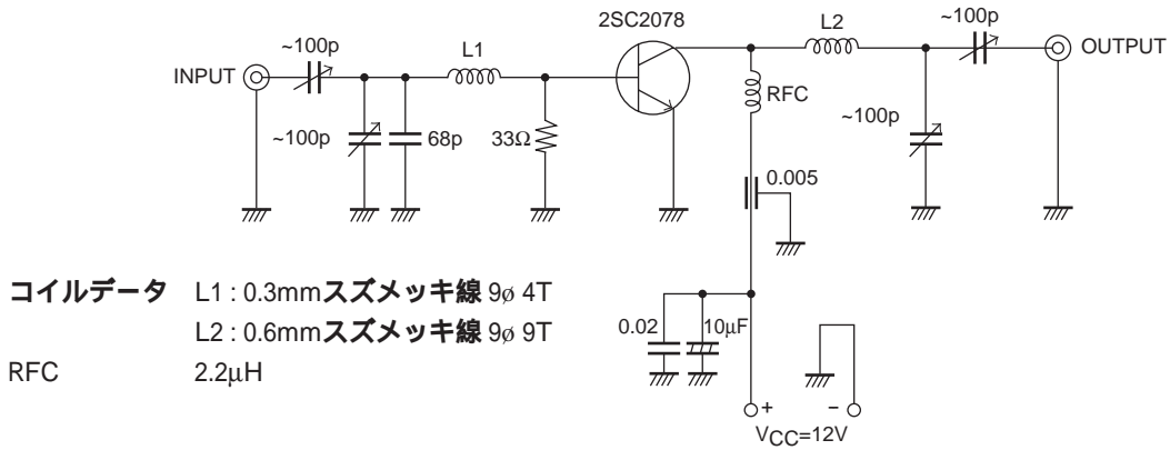
2SC2078 27MHz 出力電力測定回路図
